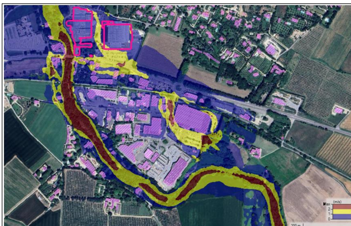
Figure 80 : Vitesses des écoulements (en m/s) pour l'état actuel – Q100 (source : Etude hydraulique OTEIS)
